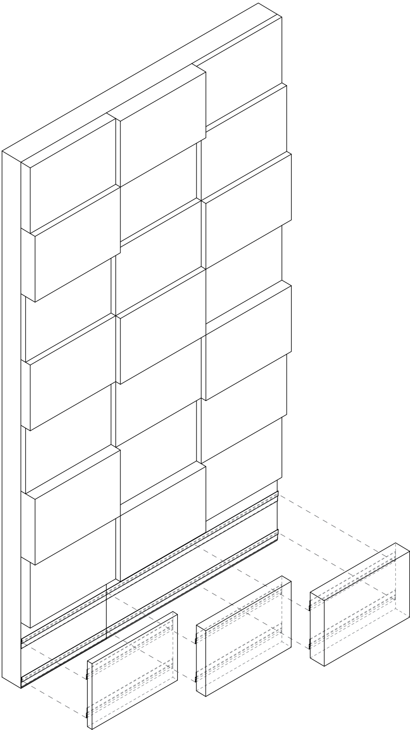
1 Muro Plus Axonometric Scale: Not to scale
