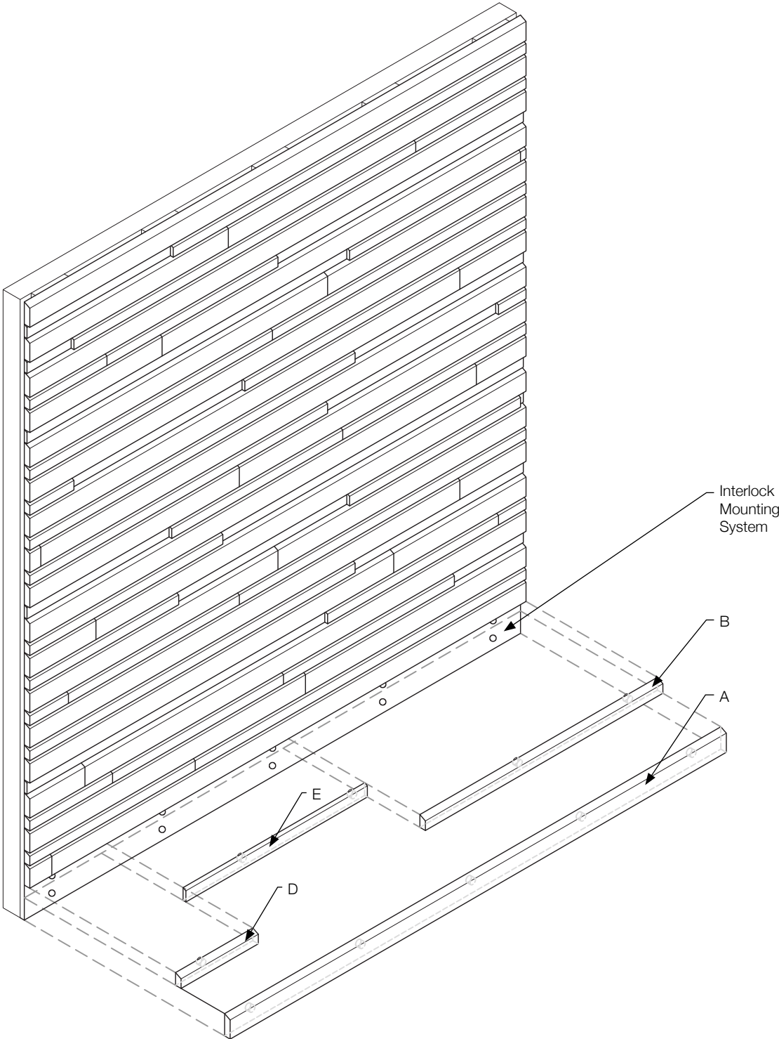
2 Exploded Axonometric Scale: 1/2" = 1'-0"
